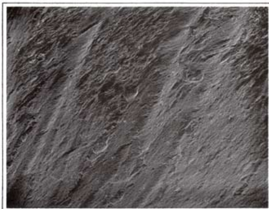
Ecaillagement op een silexartefact uit de concentratie "Eemster" van Vermaing. Vergroting: 80 \times 45^\circ . (Electronen microscoop). Geen stof of splinters waar te nemen.
