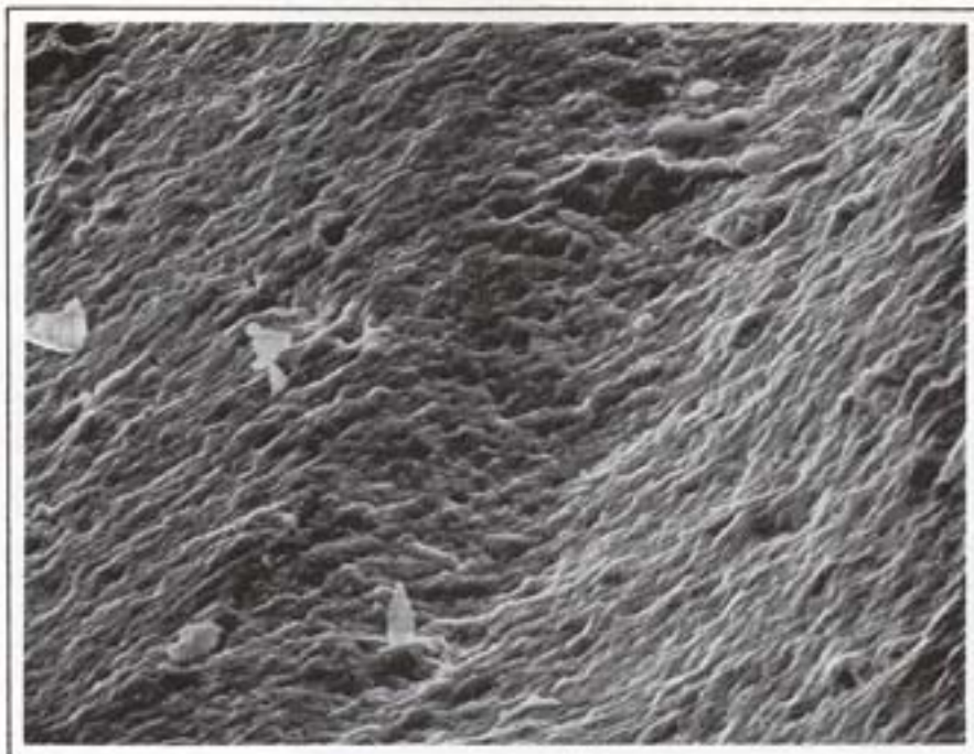
Ecaillagement op de zelfde silexafslag uit "Eemster". Het zwart omkaderde deel van de vorige foto werd gefotografeerd. Vergroting: 640 \times 45^\circ . (electr. microscoop) Geen stof. De enkele spintertjes zijn duidelijker te zien. De lichtreflectie van deze stukjes zouden de dofheid tijdelijk veroorzaken?.
